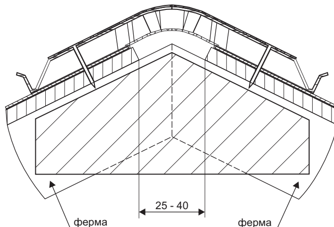
Рис. 12 Крыша из стропильных ферм
