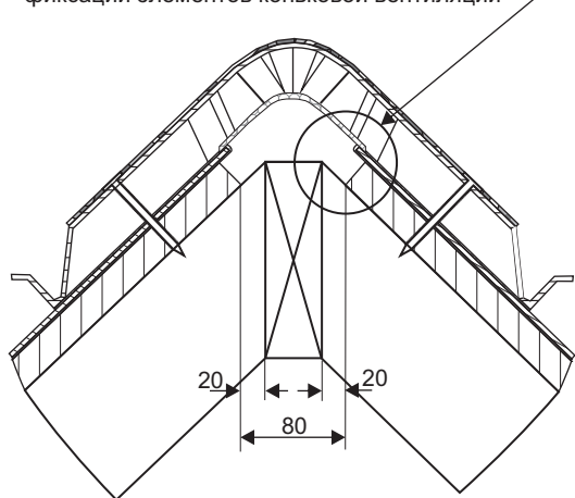
Рис. 11 Крыша с крутым уклоном (55°)
